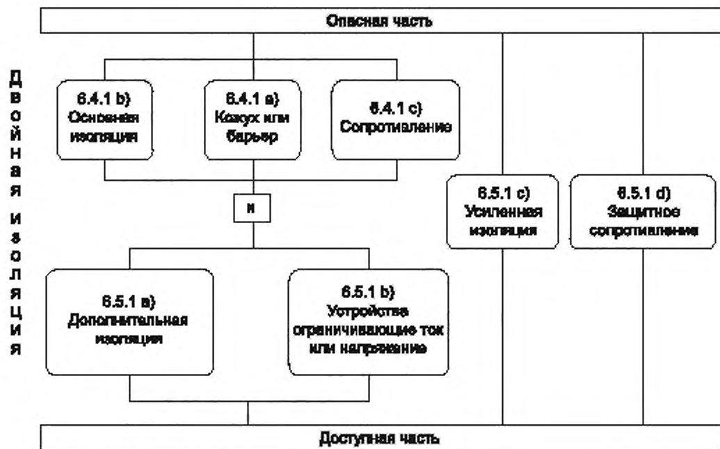
Рисунок 4 — Возможные комбинации средств защиты от поражения электрическим током
