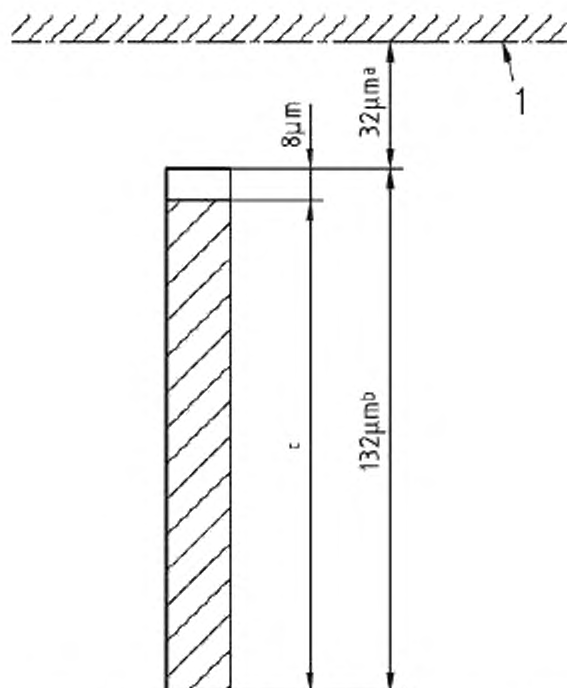
1 – нулевая линия; a – величина основного отклонения g ; b – величина допуска степени точности 6; c – уменьшенный допуск степени точности 6
