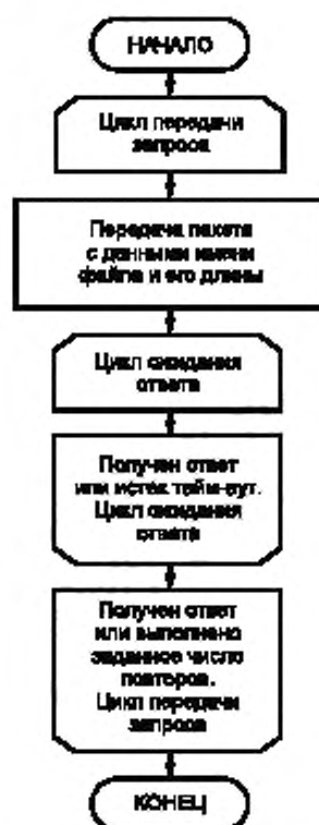
Рисунок 6 — Блок-схема алгоритма процесса запроса на передачу файла и ожидания ответа
