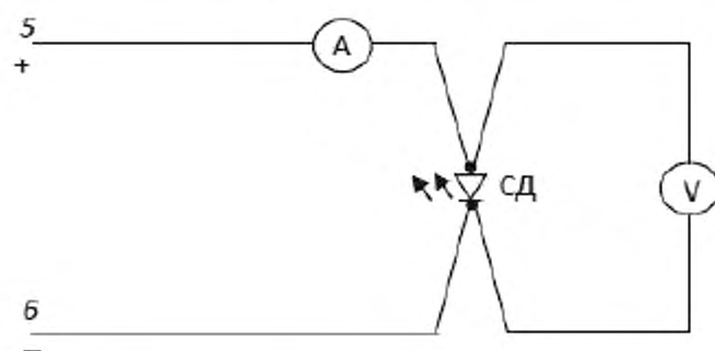
5, 6 – выводы для подключения системы питания (см. приложение А); V – вольтметр для измерения напряжения питания; A – амперметр для измерения тока лампы; СД – измеряемый светодиод
