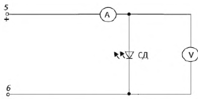
5, 6 – выводы для подключения системы питания (см. приложение А); V – вольтметр для измерения напряжения питания; A – амперметр для измерения тока СД; СД – измеряемый светодиод
