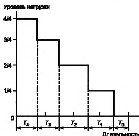
Рисунок С.3 — Пример графика длительности нагрузки
