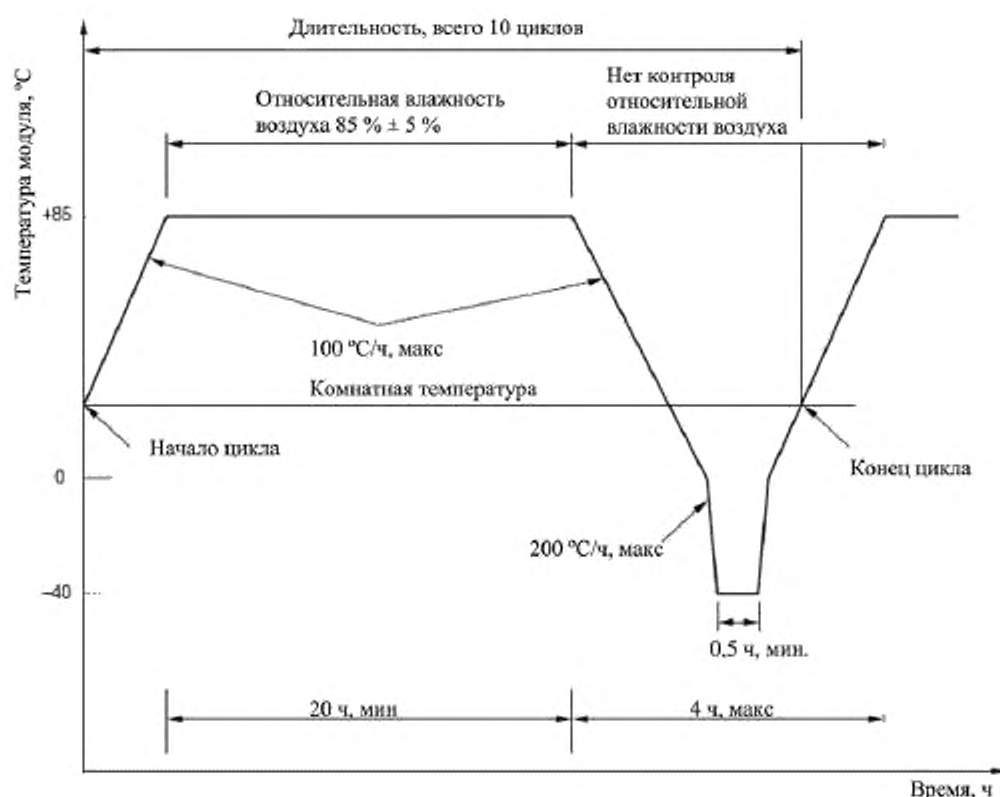
Рисунок 5 — Термоциклирование при высокой влажности
