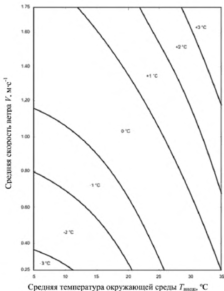
Рисунок 2 — Поправка НРТ
