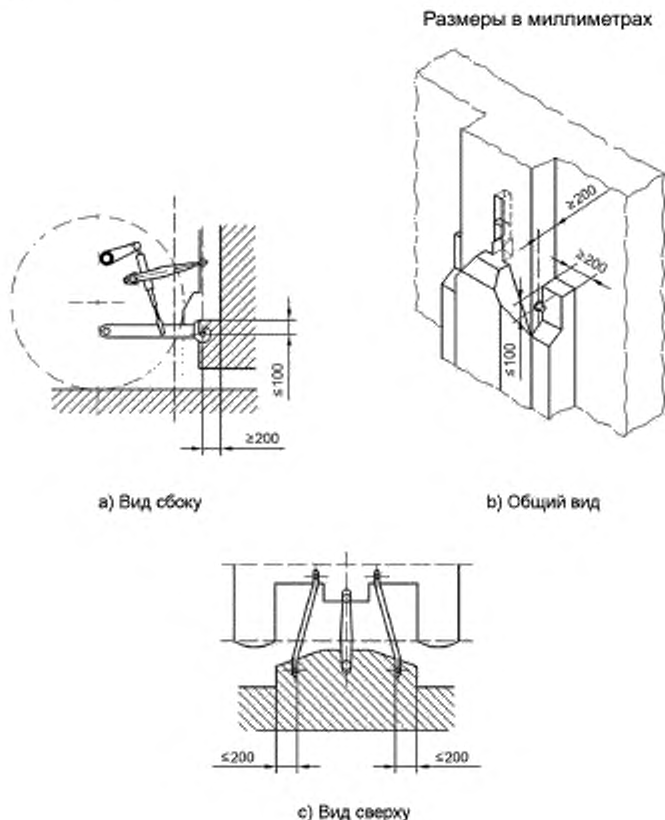
Рисунок 2 — Зона сцепления
