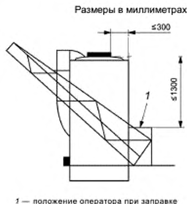
Рисунок 1 — Максимальные расстояния при ручной заправке резервуара химическими веществами
