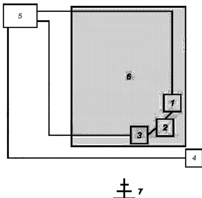
1 — АКТИВНАЯ ПРИНАДЛЕЖНОСТЬ; 2 — нагрузка; 3 — НЭ или губка, вымоченная в солевом растворе; 4 — ножной выключатель; 5 — ВЧ ЭЛЕКТРО-ХИРУРГИЧЕСКИЙ АППАРАТ; 6 — непроводящий стол; 7 — антенна — расстояние 10 м, вертикальная поляризация
