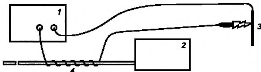
1 — ВЧ ЭЛЕКТРОХИРУРГИЧЕСКИЙ АППАРАТ; 2 — испытываемый блок; 3 — металлическая пластинка; 4 — шнур ПРИНАДЛЕЖНОСТИ испытываемого блока
