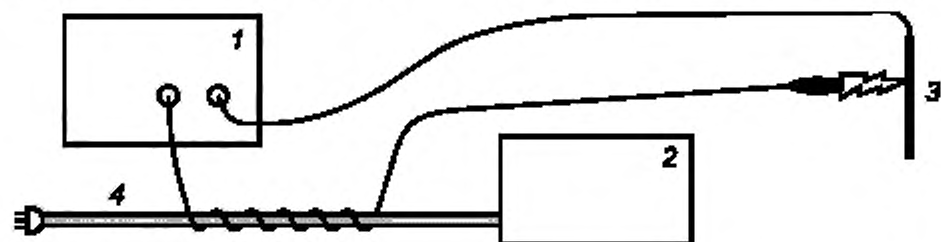
1 — ВЧ ЭЛЕКТРОХИРУРГИЧЕСКИЙ АППАРАТ; 2 — испытываемый блок; 3 — металлическая пластинка; 4 — сетевой шнур питания испытываемого блока
