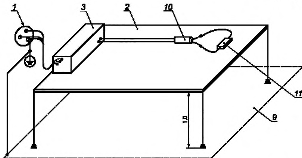
1 — ПИТАЮЩАЯ СЕТЬ; 2 — стол, изготовленный из изолирующего материала; 3 — ВЧ ЭЛЕКТРОХИРУРГИЧЕСКИЙ АППАРАТ, 9 — заземленная проводящая поверхность. 10 — активированный БИПОЛЯРНЫЙ ЭЛЕКТРОД , 11 — требуемое сопротивление нагрузки с устройством измерения ВЧ мощности
