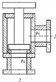
Рисунок 1 — Угловой клапан
