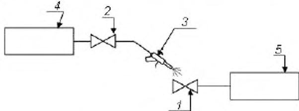
1 — испытуемый клапан, 2 — клапан, 3 — обдуватель, 4 — резервуар с пробным газом, 5 — система течеискателя
