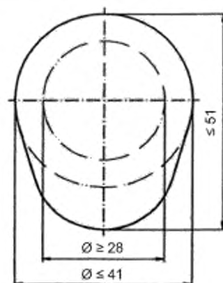
Рисунок 2 — Профиль жерди
