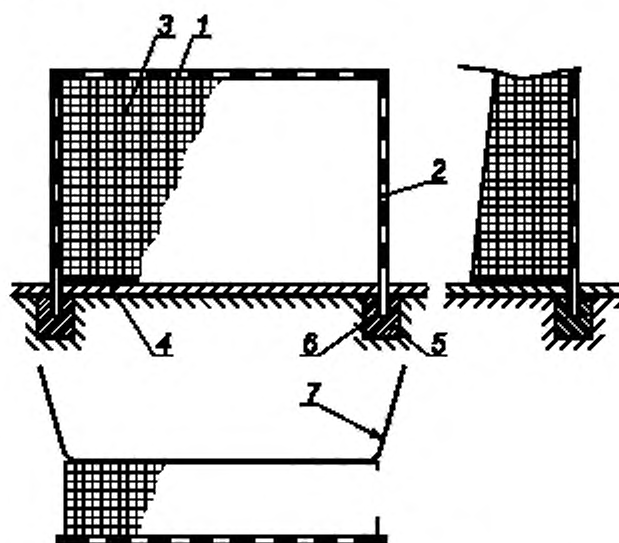
1 — перекладина; 2 — штанги; 3 — сетка; 4 — планка натяжения сетки; 5 — бетон; 6 — установочные гильзы; 7 — шнур натяжения сетки
