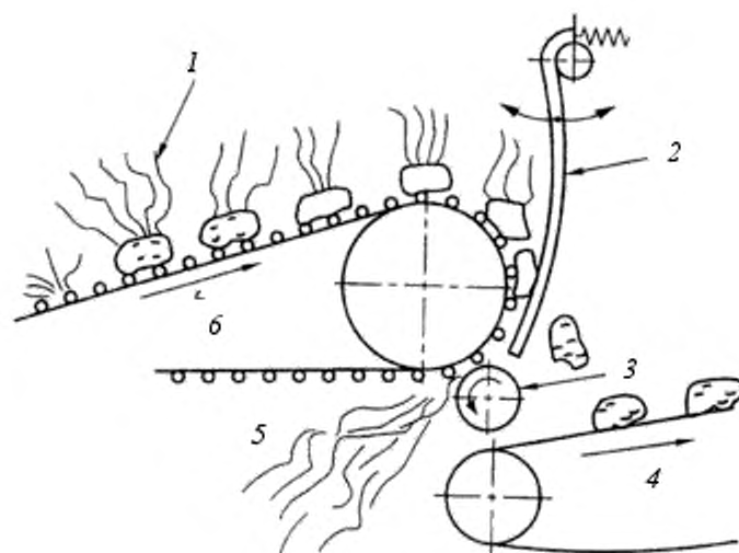
1 – ботва, 2 – пальцы для отделения ботвы, 3 – ролики для отделения ботвы, 4 – цепь конвейера, 5 – выброс ботвы, 6 – подъемная цепь
