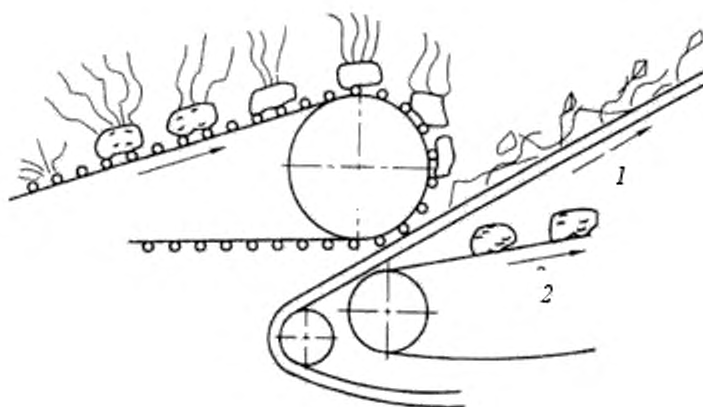
1 – цепь для отделения ботвы, 2 – цепь конвейера
