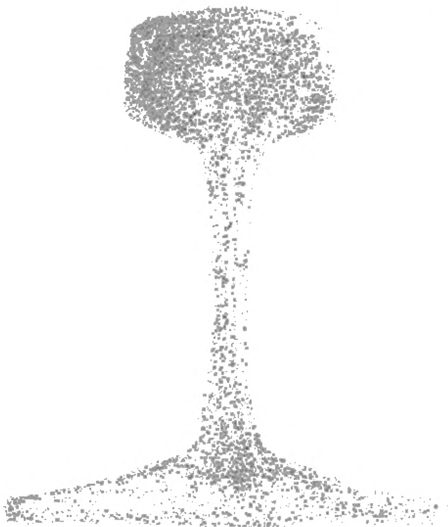
Рисунок И.3 — Обратная ликвация в шейке (серый отпечаток)
