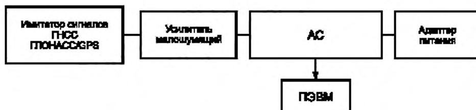
Рисунок Д.1 — Схема испытательного стенда
