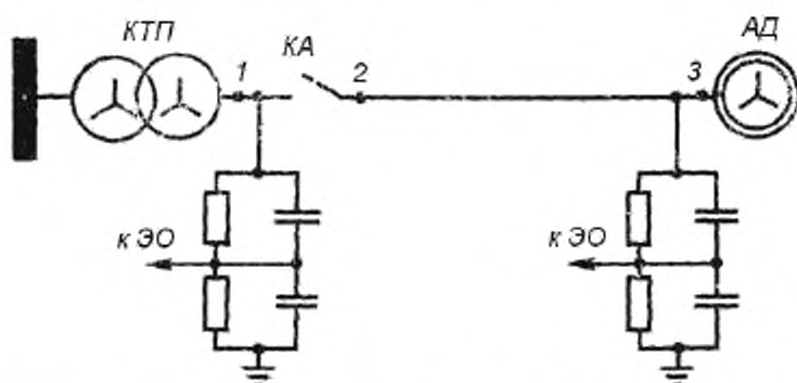
Схема коммутации низкого напряжения
