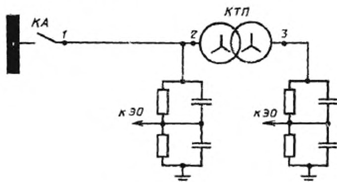
Схема коммутации низкого напряжения
