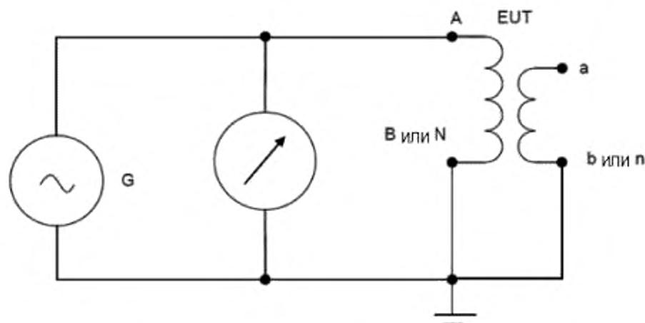
EUT — объект испытания, G — испытательный генератор напряжения
