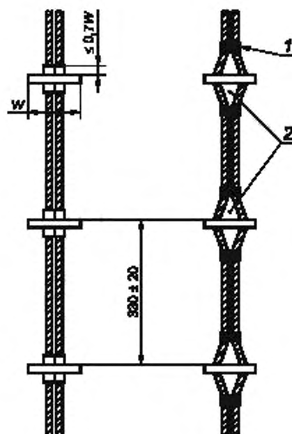
1 — бензель (типовой); 2 — клинья
