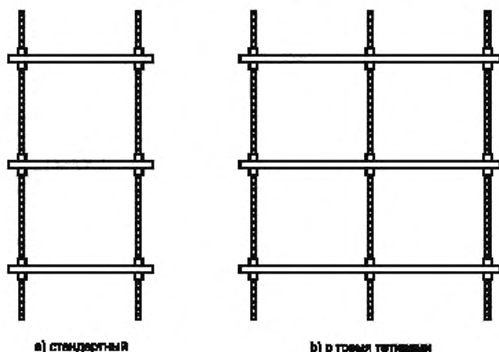
Рисунок 1 — Штурмтрапы
