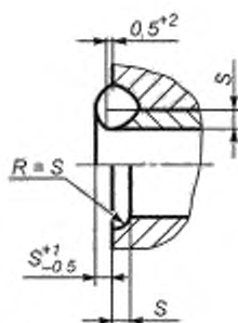
Рисунок 8 — Сварное соединение типа C2
