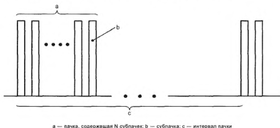
Рисунок 7 — Радиointерфейс DSSS
