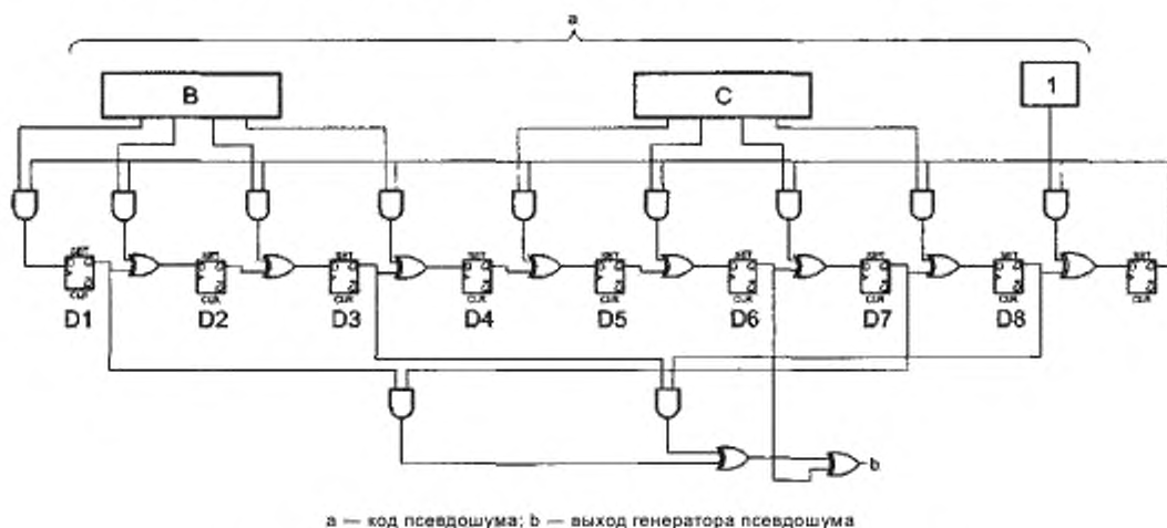
Рисунок 5 — Генератор псевдoshума передатчика электронной пломбы
