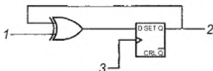
1 — вход данных; 2 — выход данных из; 3 — тактовый сигнал
