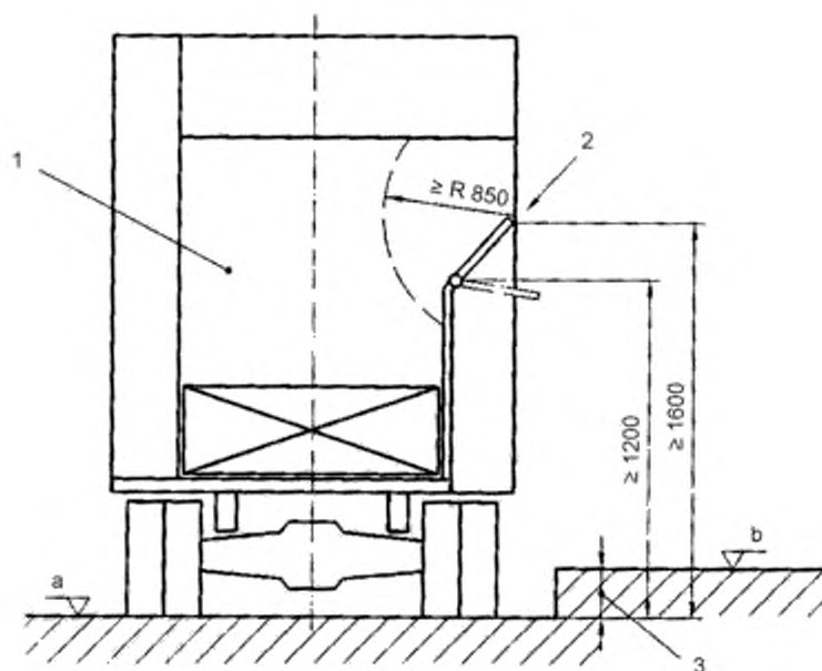
1 – бункер; 2 – силовая балка; 3 – стандартная высота бордюра, равная 200 мм; а – уровень стоянки мусоровоза; б – бордюр
