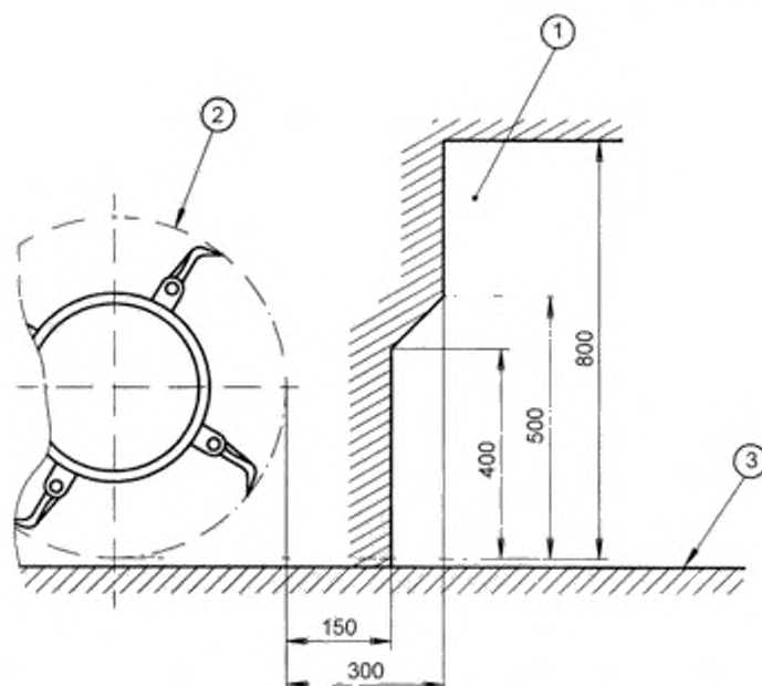
1 – зона внутри ограждения (отражательная пластина); 2 – траектория движения рабочего органа; 3 – почва
