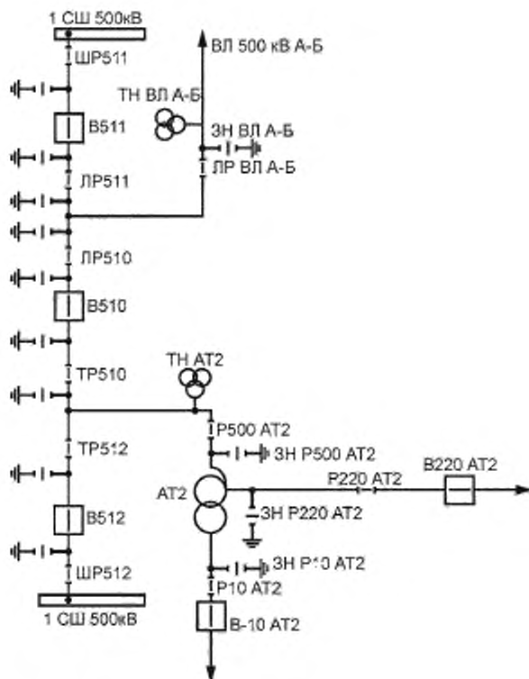
Рисунок Е.3 — Схема ПС 500 кВ, выполненная по полупотрону схеме
