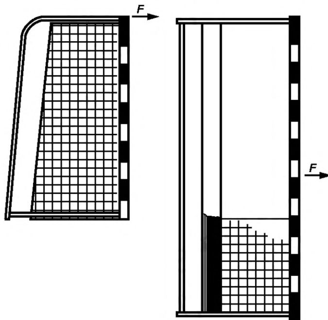
Рисунок 12 — Проверка стабильности ворот для мини-футбола
