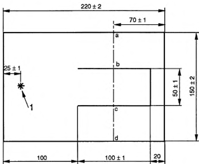
Рисунок 2 – Испытуемый образец в форме языка
