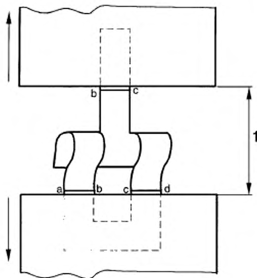
Рисунок 3 — Расположение зажимов
