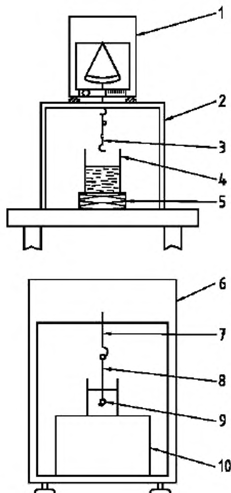
1 — весы; 2 — опорная рама; 3 — проволоочная подвеска; 4 — лабораторный стакан; 5 — подставка для стакана; 6 — весы; 7 — крюк для подвешивания; 8 — проволоочная подвеска; 9 — образец для испытаний; 10 — опорная подставка
