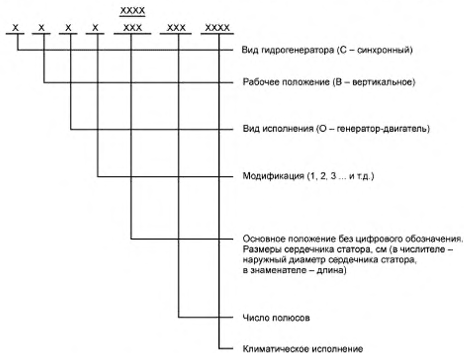
Рисунок А.1 — Структура условного обозначения гидрогенератора
