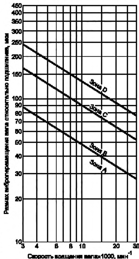
Рисунок A.1 — Рекомендуемые значения максимальных относительных перемещений вала в зависимости от максимальной рабочей скорости вращения вала агрегата
