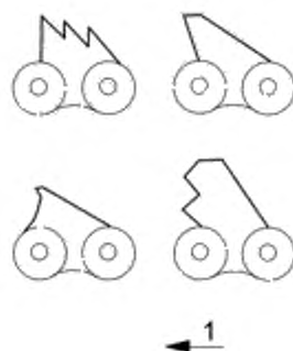
Рисунок С.4 – Вид сбоку неприемлемого профиля зуба цепи
