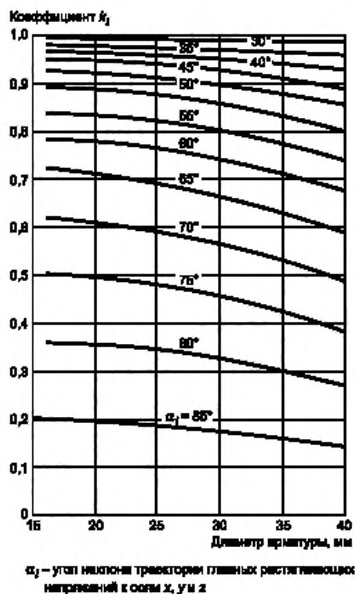
Рисунок Д.1 — Номограмма для определения коэффициента K_1
