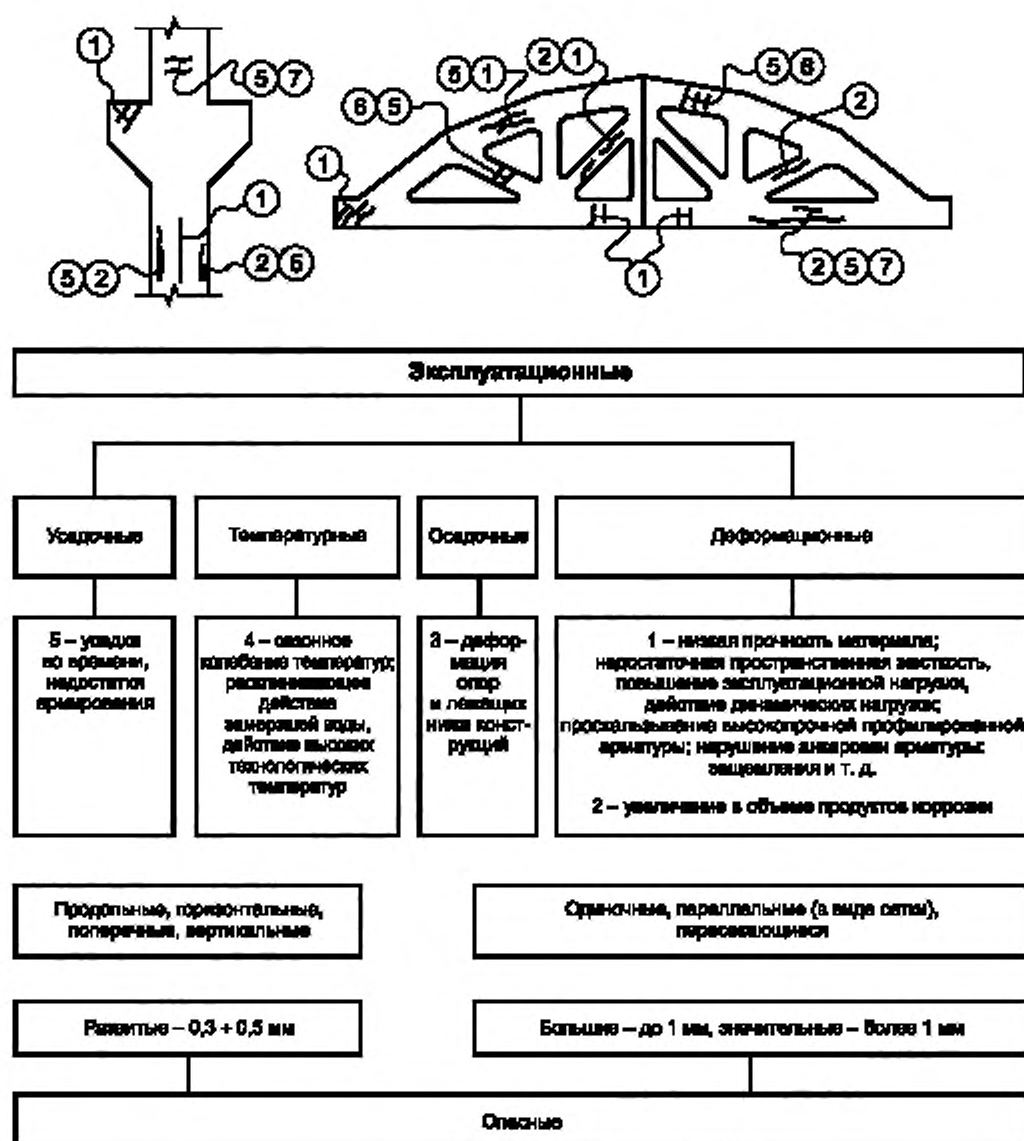
Рисунок К.2 — Эксплуатационные виды трещин
