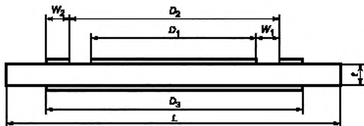
Рисунок 24 — Электроды для измерений объемного и поверхностного сопротивления
