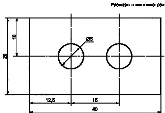
Рисунок 35 — Образец для проведения испытаний на сопротивление изоляции
