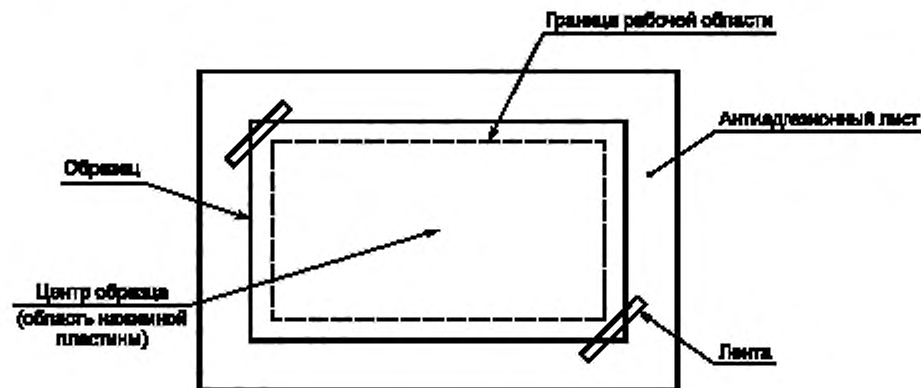
Рисунок 16 — Схема расположения образца перед прессованием
