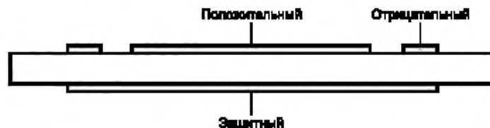
Рисунок 26 — Подсоединения электродов для измерения поверхностного сопротивления
