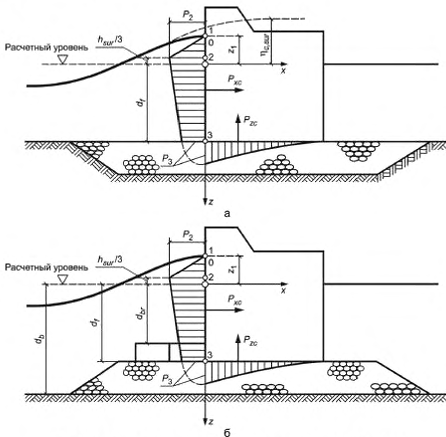
Рисунок 9 — Эпюры давления прибойных волн на вертикальную стену
