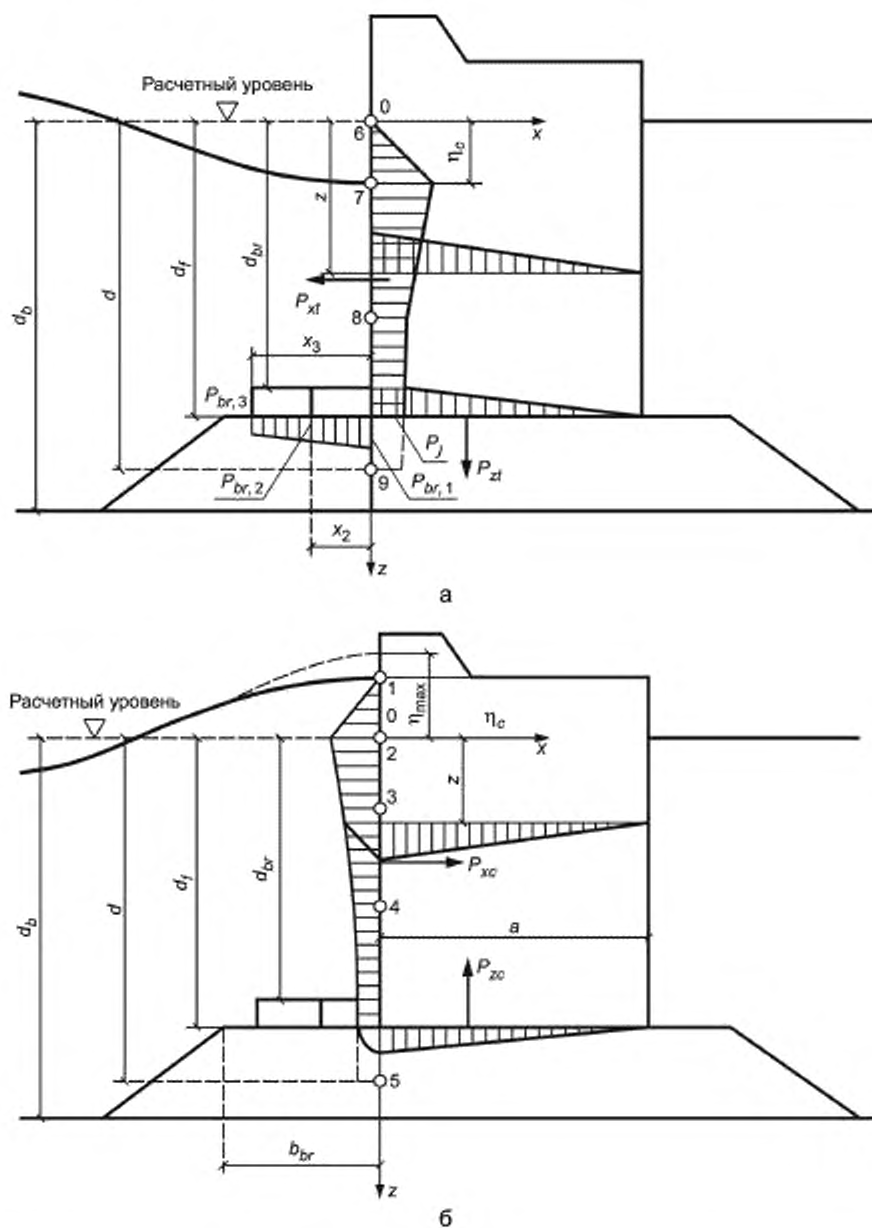
Рисунок 1 — Элюры давления стоячих волн на вертикальную стену со стороны открытой акватории
