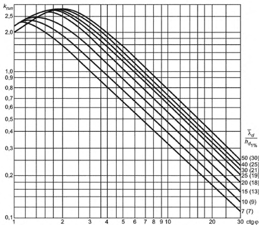
Рисунок 10 — Графики значений коэффициента k_{nm}
