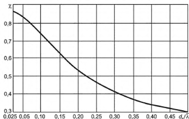
Рисунок 32 — График значений коэффициента \chi
