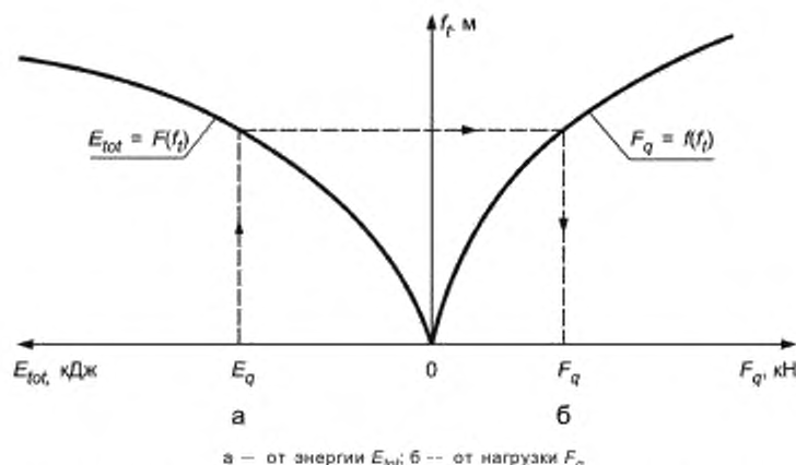
Рисунок 33 — Схема построения графиков зависимости деформаций отбойного устройства (и причального сооружения) f_i
