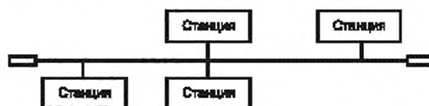
Рисунок 5 — Топология «шина»
