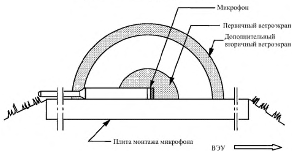
Рисунок 1б – Монтаж микрофона (вид сбоку)
