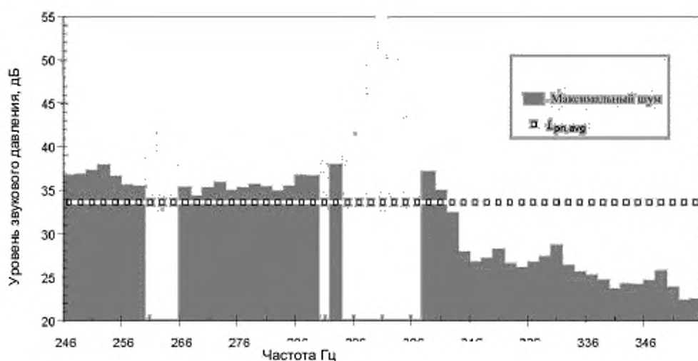
Рисунок 10 – Иллюстрация уровня L_{p1,avg} и линий, классифицируемых как маскирующие
