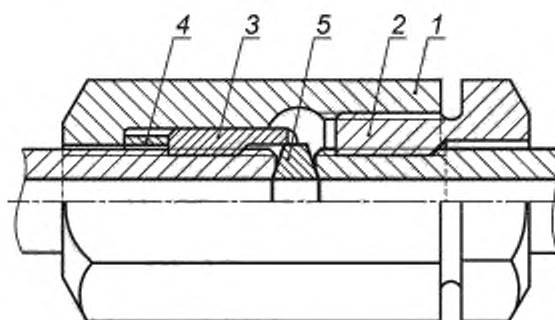
1 — гайка накидная; 2 — втулка резьбовая; 3 — гайка упорная; 4 — контргайка; 5 — линза по ГОСТ 10493
