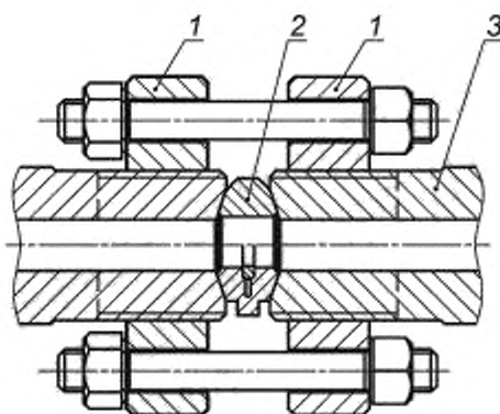
1 — фланец резьбовой по ГОСТ 9399; 2 — линза по ГОСТ 10493, 3 — конец трубы присоединительный резьбовой по ГОСТ 9400
