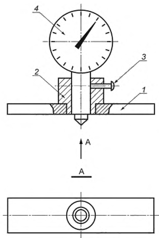
1 — пластина; 2 — втулка; 3 — винт; 4 — индикатор часового типа
