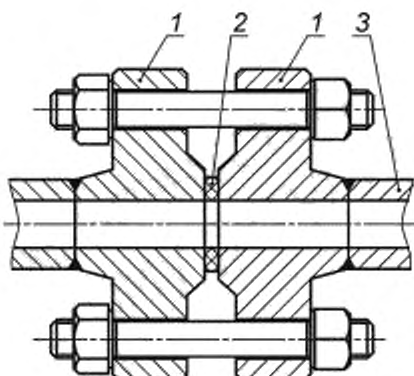
1 — фланец по ГОСТ Р 54432; 2 — прокладка; 3 — труба
