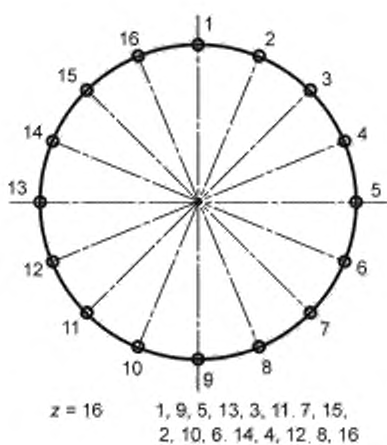
Рисунок М.2 — Схемы перестановки ключа при затяжке шпилек разъёмных соединений с различным количеством шпилек z
