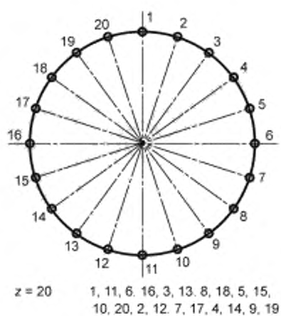
Рисунок М.2 — Схемы перестановки ключа при затяжке шпилек разъёмных соединений с различным количеством шпилек z
