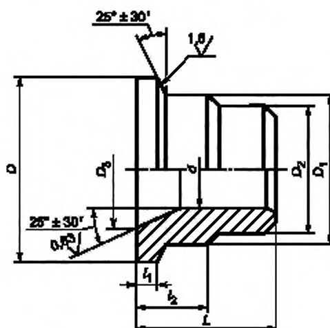
Рисунок 5 — Приварной ниппель
