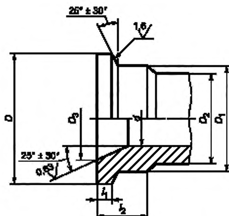
Рисунок 6 — Ниппель неприварной
