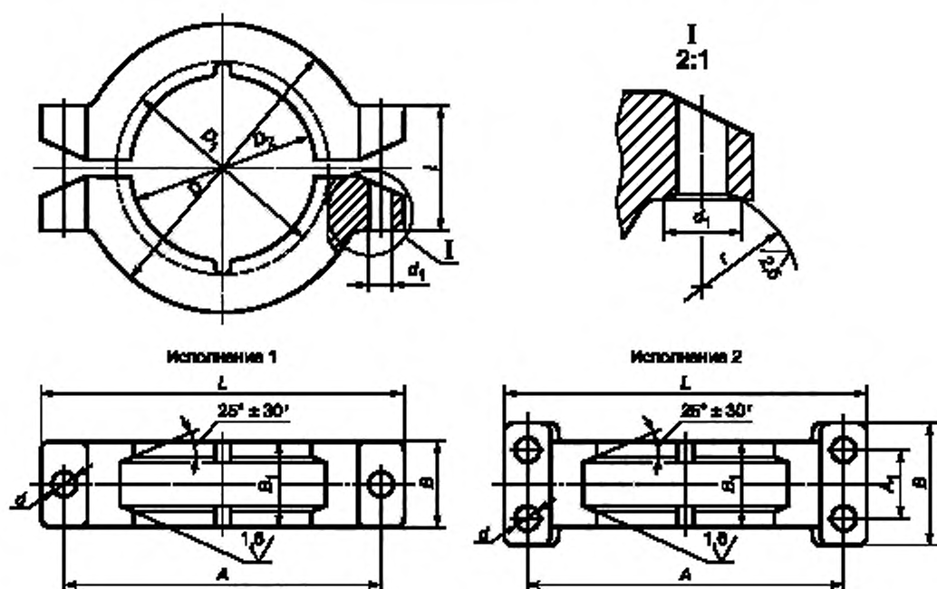
Рисунок 2 — Бугель
