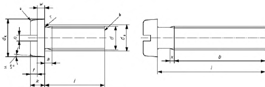
Рисунок 1 — Винт с низкой цилиндрической головкой со шлицем
