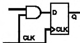
Связь сигнала данных с синхросигналом
