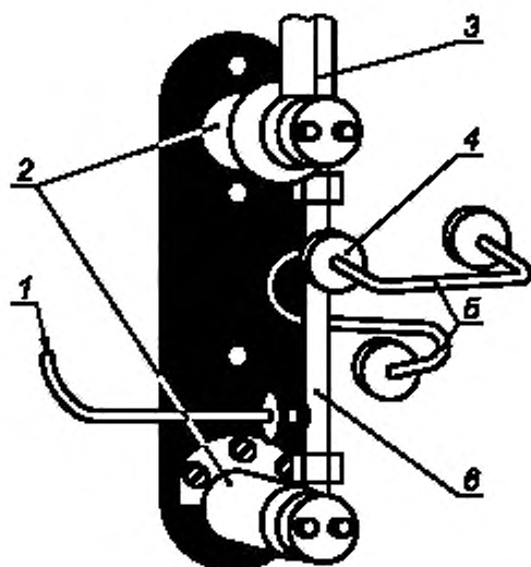
1 — впуск топлива; 2 — охлаждаемые шины; 3 — термодатчик; 4 — испытательный фильтр; 5 — выпуск топлива; 6 — испытательная секция нагревателя
