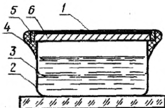
1 — испытуемый слой СФТК; 2 — стеклянная чаша; 3 — дистиллированная вода; 4 — герметизирующая мастика; 5 — слой парафина; 6 — подложка (утеплитель)
