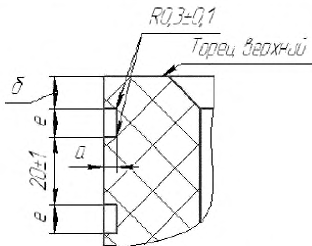
Рисунок А.14 — Конструкция канавки под уплотнительные прокладки на верхнем торце царг типа ЦНК, ЦНКО
