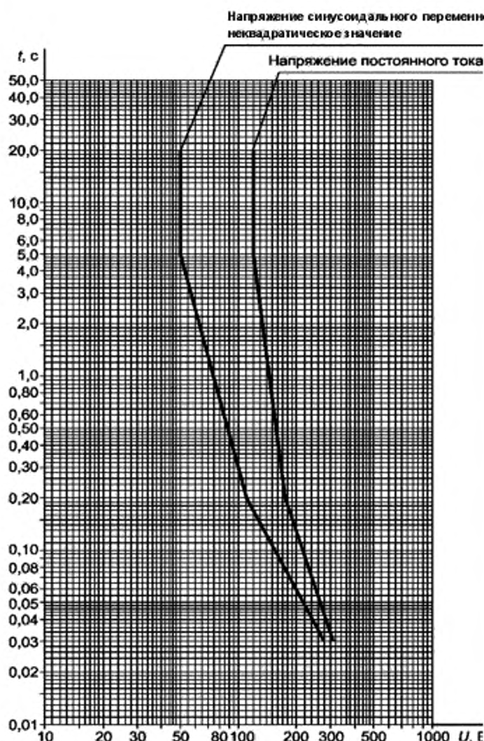
Рисунок 1 — Максимальное допустимое время, в течение которого доступная часть может находиться под кратковременным изредка появляющимся на доступной части напряжением в условиях одной неисправности (см. 6.3.2.1)
