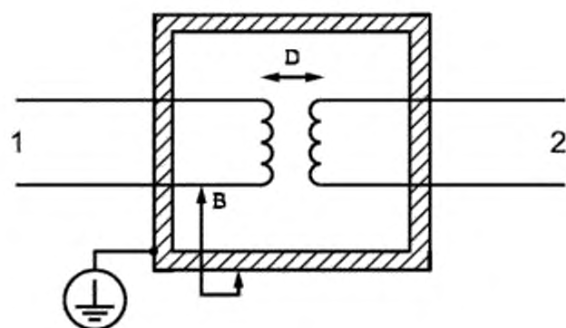
1 — опасная цепь; 2 — безопасная цепь
