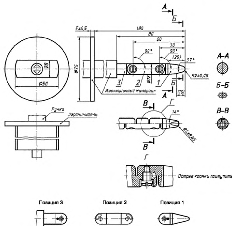
Рисунок В.2 · Шарнирный испытательный палец
