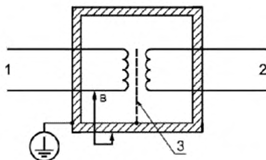
1 — опасная цепь; 2 — безопасная цепь; 3 — защитный экран
