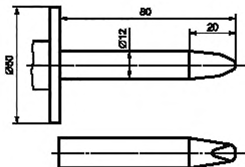
Рисунок В.1 — Жесткий испытательный палец (испытательный щуп по стандартам государства )
