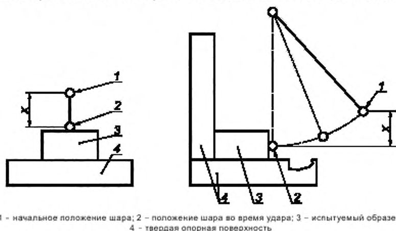
Рисунок 4 — Испытание на удар с помощью шара
