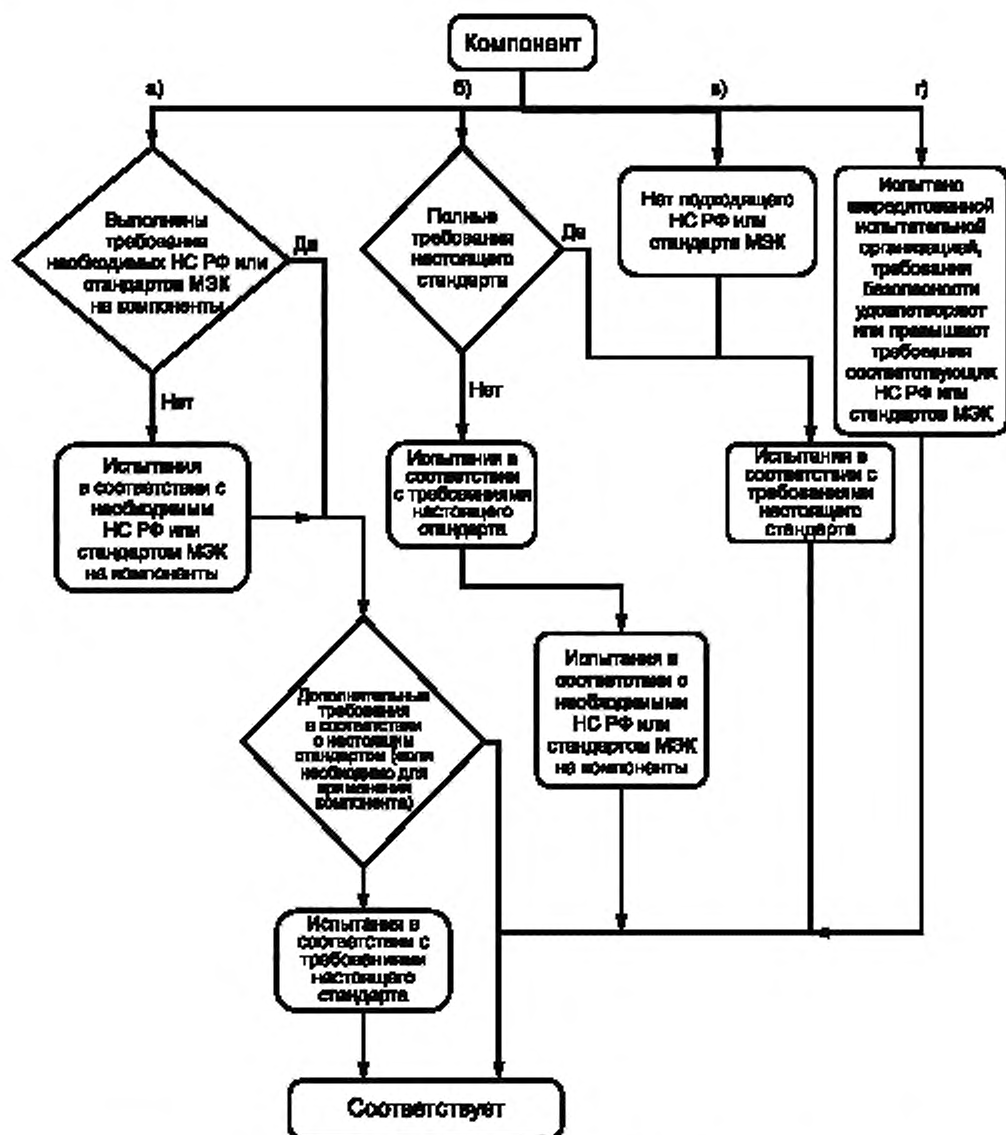
Рисунок 10 — Блок-схема для вариантов соответствия по 14.1, перечисления а), б), е) и г)
