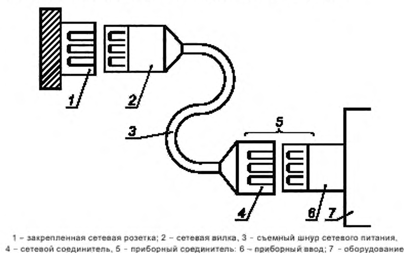
Рисунок 3 – Съемные шнуры сетевого питания и соединители
