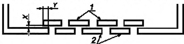
Рисунок 6 – Перегородки
