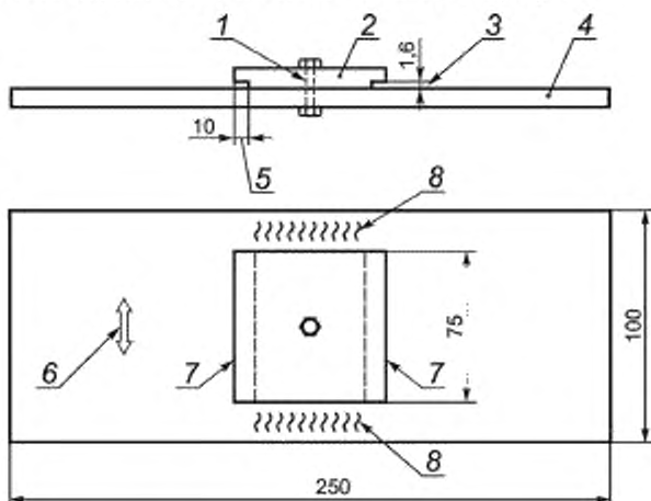
1 — отверстие диаметром 13 мм; 2 — верхняя плита; 3 — зазор в корневом вырезе; 4 — нижняя плита; 5 — глубина корневого выреза; 6 — предпочтительное направление прокатки; 7 — испытываемые швы; 8 — крепежные швы
