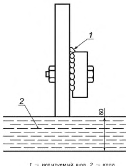
1 — испытуемый шов. 2 — вода
