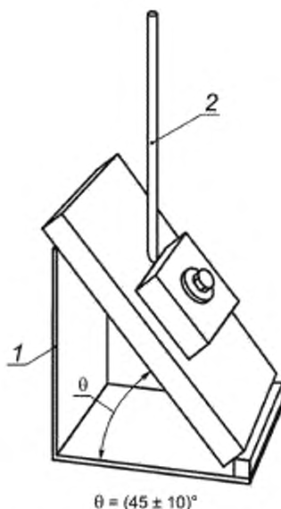
1 – приспособление для проведения испытания, 2 – сварочный материал
