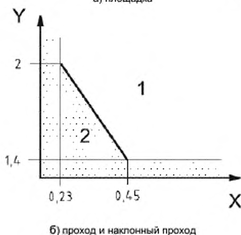
Рисунок 12 – Связь между высотой в свету и шириной площадки или прохода
