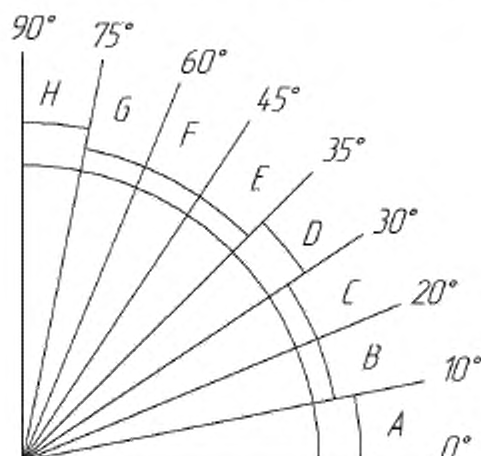
А — пандус рекомендуемый; В — пандус с повышенным сопротивлением скольжению; С — лестница с углом наклона от 20° до 30°; D — лестница с углом наклона от 30° до 38°, рекомендуемая; E — лестница с углом наклона от 38° до 45°; F — лестница с углом наклона от 45° до 60°, рекомендуемая; G — лестница с углом наклона от 60° до 75°; H — лестницы крутонаклонные и вертикальные рекомендуемые
