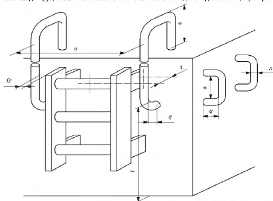
о – длина поручня для захвата рукой; n – диаметр/ширина поручня; q – зазор для размещения руки (между поручнем и монтажной поверхностью); f – вертикальное расстояние между нижней частью поручня и полом/настилом; s – вертикальное расстояние между верхней частью поручня и настилом площадки, расположенной в верхней части лестницы; f2 – зазор между краем поручня, расположенного вдоль лестницы, и краем ступени/тетивы лестницы; u – расстояние между параллельными поручнями, между которыми должен быть обеспечен проход; z – расстояние между ступенью и поручнем
