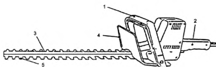
1 — передняя рукоятка; 2 — задняя рукоятка; 3 — режущий механизм; 4 — ограждение; 5 — зуб режущего лезвия
