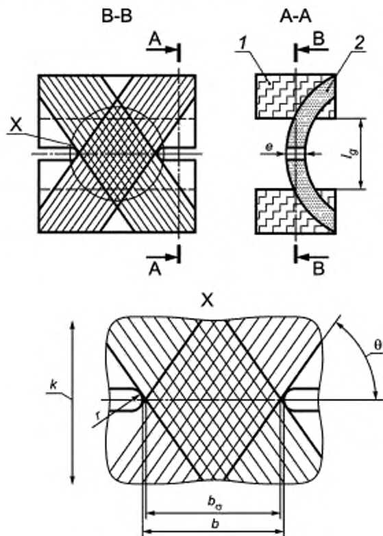
Рисунок 9 — Схема крепления образца (метод Е)
