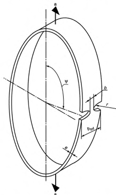
Рисунок 4 — Образец для испытания (метод Б)
