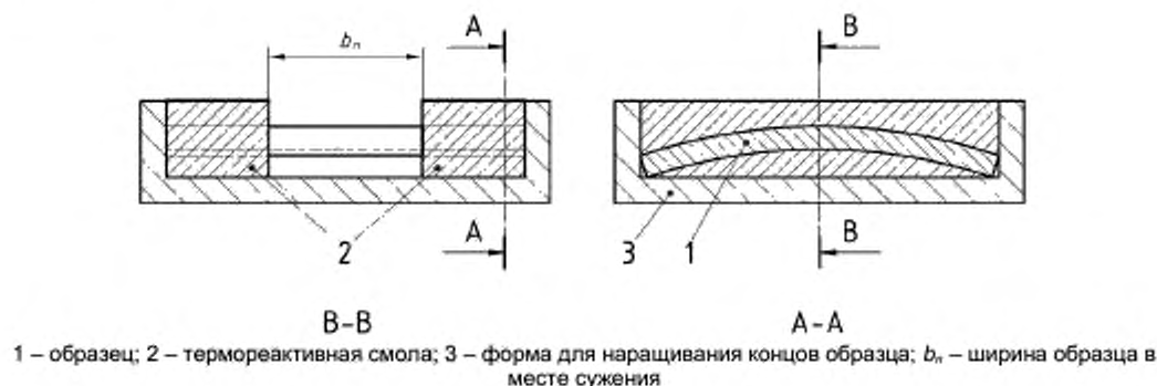
Рисунок 5 – Наращивание термореактивной смолой на сторонах образца
