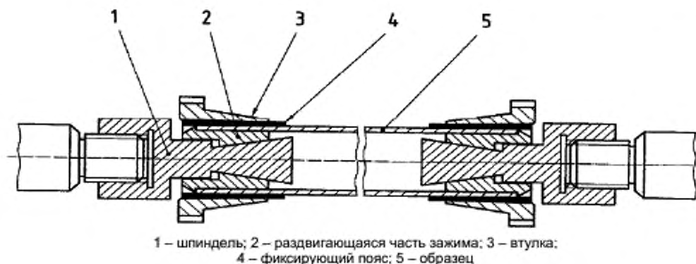
Рисунок 1 – Зажим для крепления образца (для метода Б)
