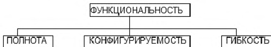
Рисунок 2 — Иерархия функциональности
