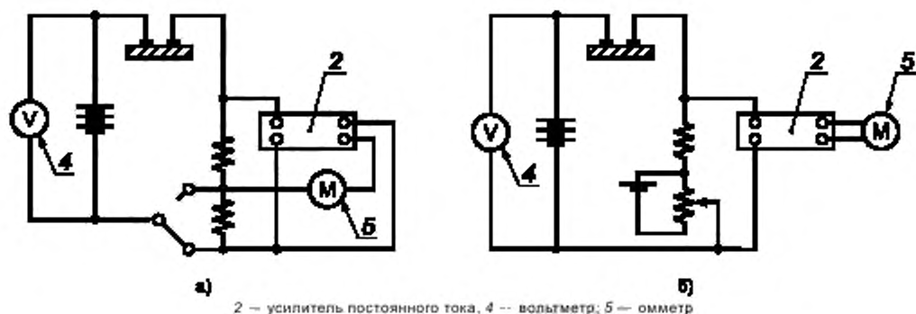
2 — усилитель постоянного тока; 4 — вольтметр; 5 — омметр
