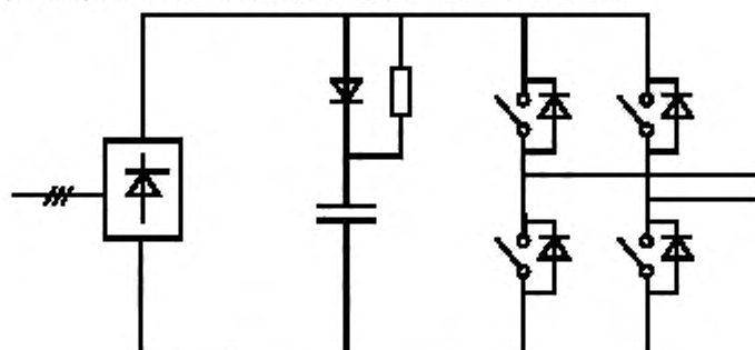
Рисунок С.4 — Снаббер в звене постоянного тока
