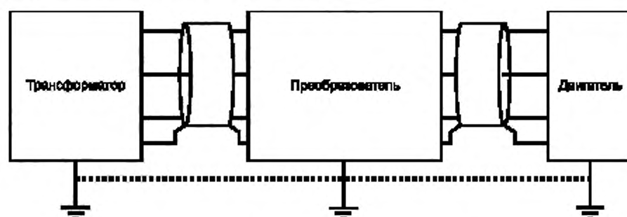
Рисунок 22 — Пример защитного заземления и соединения основных компонентов
