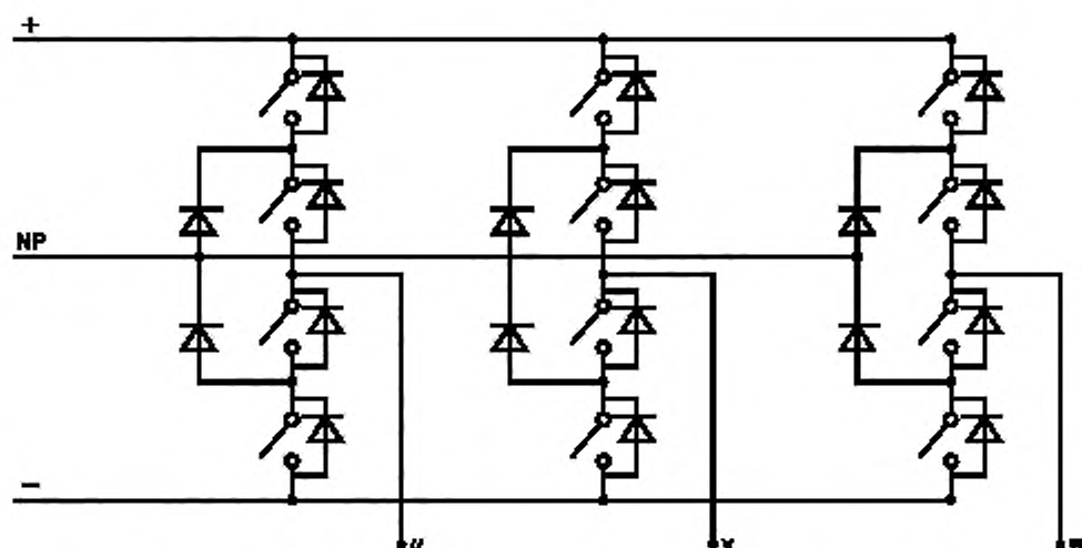
Рисунок А.7 — Схема инвертора с выведенной нейтралью
