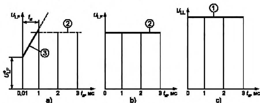
Рисунок 19 — Допустимые импульсные напряжения (с учетом отражения и демпфирования) на зажимах двигателя в функции времени нарастания t_F пика напряжения определяются (цифры на рисунке являются общими ссылками для рисунка 17 и таблицы 7): а) межвитковой изоляцией и конструкцией обмотки; б) основной изоляцией между обмоткой и корпусом; в) основной межфазной изоляцией.
