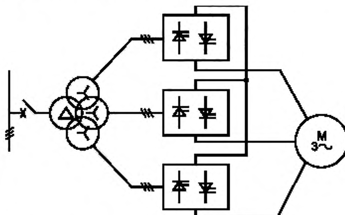
Рисунок A.14 — Трехфазный шестипульсный циклоконвертер с четырехобмоточным трансформатором
