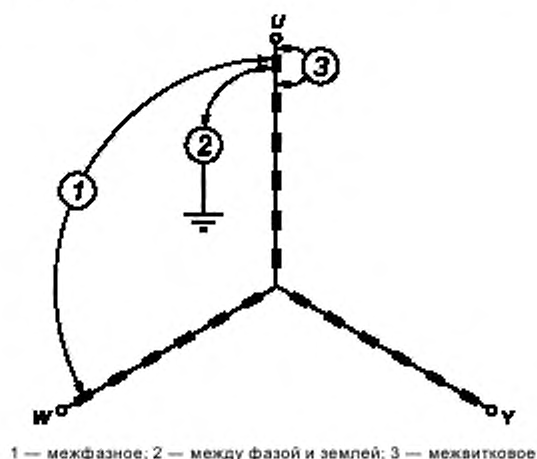
Рисунок 17 — Виды перенапряжений на изоляции
